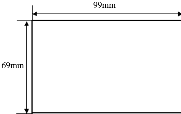
图 2-2 外引键盘安装尺寸
